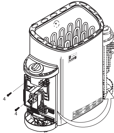
그림 5B | 부착형 컨트롤유닛의 재배치 Fig. 5B | Repositioning the Built-in-Control Unit
