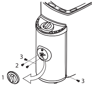
그림 5A | 컨트롤유닛의 개봉 Fig. 5A | Opening of the Control Unit
