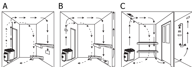
그림 7 환기 Fig. 7 Air ventilation
